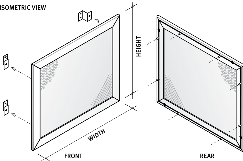
TYPE SP13
