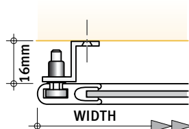
TYPE SP16
