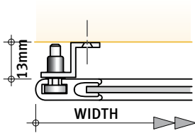
TYPE SP13
